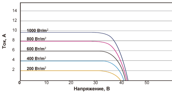
Зависимость тока и напряжения от интенсивности солнечного излучения
