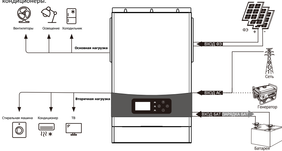
Рисунок 1. Гибридная энергосистема
