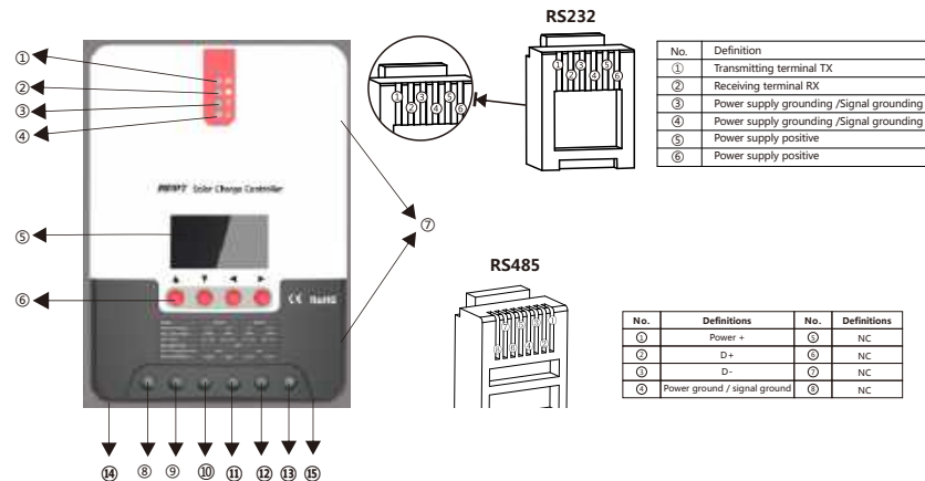
Рис. 1-1 Внешний вид и интерфейсы подключений
