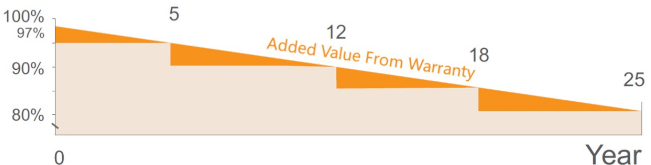
Прогнозируемое сохранение мощности солнечного модуля
