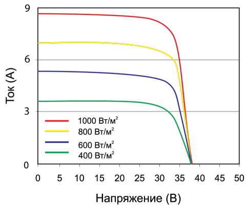
Зависимость электрических параметров от интенсивности солнечного света
