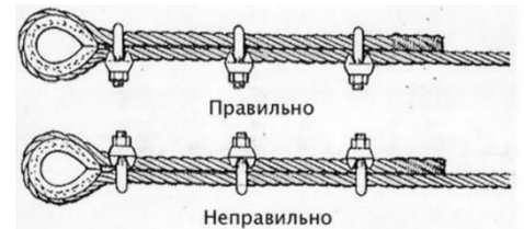
Способы крепления троса к на мачте.
