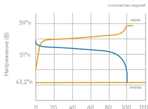
Заряд и разряд при 25°C, 0.5C
